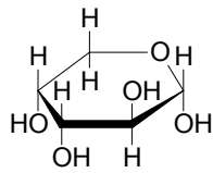
\alpha -D-Arabinopyranose
