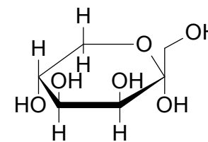
\alpha -D-Tagatopyranose
