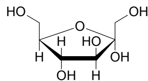
\alpha -D-Fructofuranose
