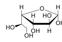
\alpha -D-Idofuranose
