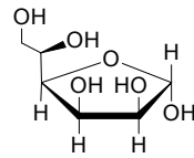
\alpha -D-Mannofuranose
