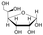
\alpha -D-Allofuranose
