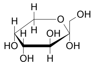
\alpha -D-Fructopyranose
