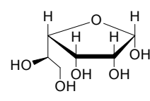
\alpha -D-Gulofuranose
