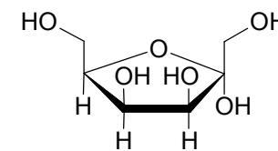
\alpha -D-Tagatofuranose
