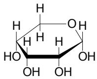
\alpha -D-Ribopyranose
