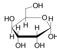
\alpha -D-Gulopyranose
