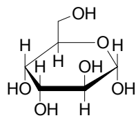
\alpha -D-Altropyranose
