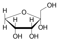
\alpha -D-Ribulofuranose
