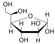
\alpha -D-Altrofuranose
