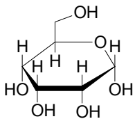
\alpha -D-Allopyranose
