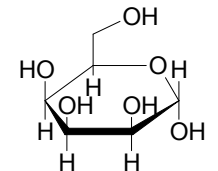
\alpha -D-Talopyranose
