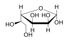
\alpha -D-Talofuranose
