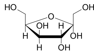
\alpha -D-Sorbofuranose
