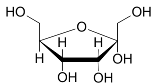
\alpha -D-Psicofuranose
